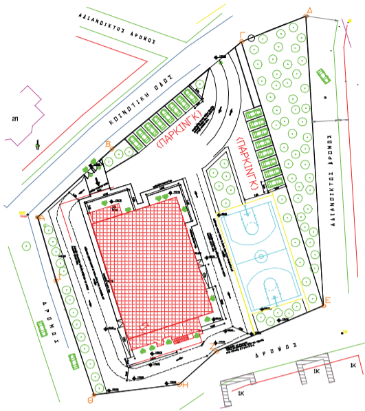
Σχέδιο διαμόρφωσης
